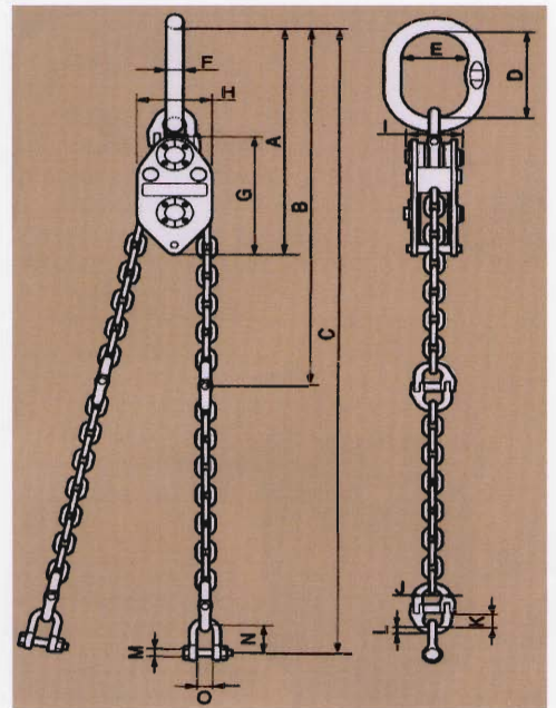
■チェーンエコライザー仕様寸法図
