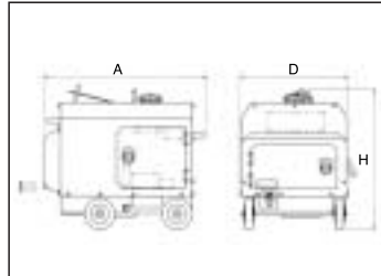
寸法図
